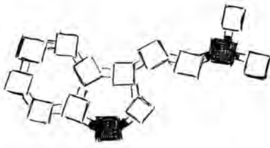
Dimethyltryptamine (DMT)
