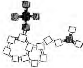
Psilocybin
