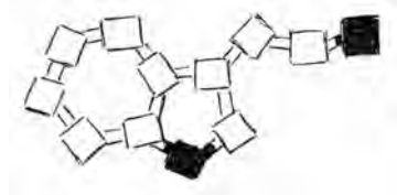
Tryptamine
